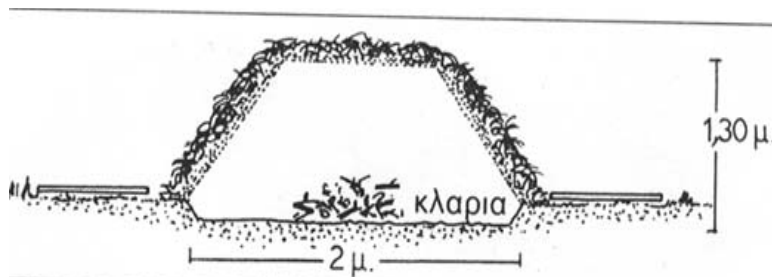
Σχήμα 3. Κάθετη τομή σωρού κομπόστ
